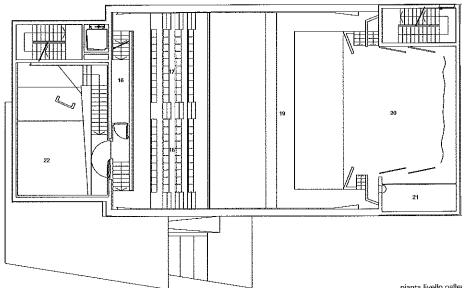
pianta livello galleria
